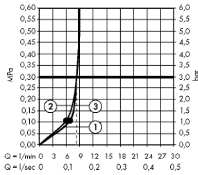
· Croma 100 Ручной душ Multi EcoSmart 9 л / мин # 28538000
