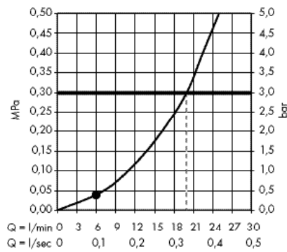
· Crometta Верхний душ 160 1jet # 26577000, 26577400
