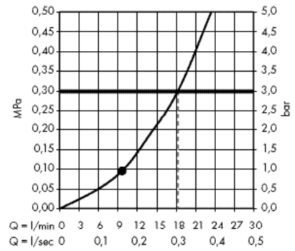
· Crometta S Верхний душ 240 1jet # 26723000
