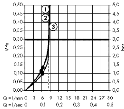
· Croma Select S Ручной душ Vario EcoSmart 9 л / МИН # 26803400
