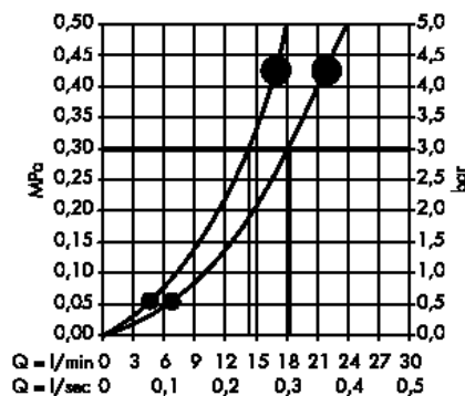
· Crometta 85 Верхний душ Vario # 28424000
