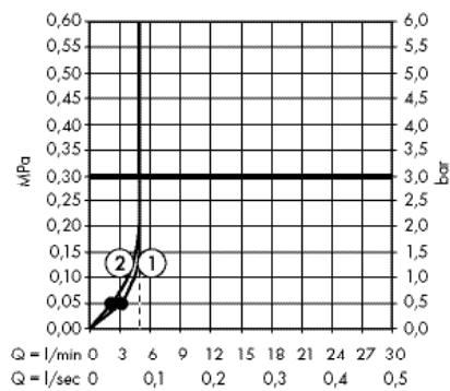
· Crometta Ручной душ Vario Green 6 л / МИН # 26336400
