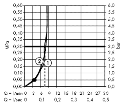
· Crometta Ручной душ Vario EcoSmart 9 л / МИН # 26332400
