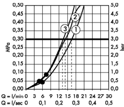
· Crometta 85 Ручной душ Multi # 28563000
