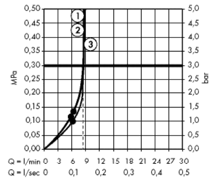
· Croma Select S Ручной душ Multi EcoSmart 9 л / мин # 26801400
