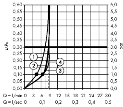
· Crometta 100 Ручной душ Vario EcoSmart 9 л / МИН # 26827400
