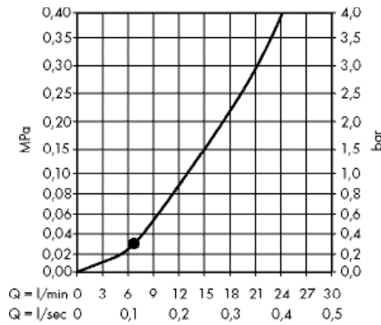
· Crometta E Верхний душ 240 1jet LowPressure # 26722000
