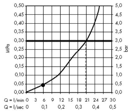
· Crometta Верхний душ 160 1jet LowPressure # 26576000, 26576400
