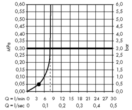
· Crometta Ручной душ 1jet EcoSmart 9 л / мин # 26333400
