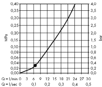
· Crometta S Верхний душ 240 1jet LowPressure # 26725000
