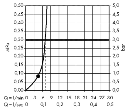
· Crometta 100 Ручной душ 1jet EcoSmart 7 л / МИН # 26829400
