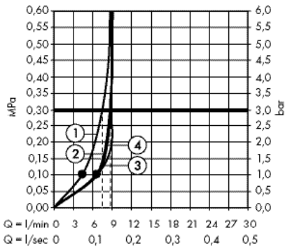
· Croma 100 Ручной душ Vario EcoSmart 9 л / мин # 28537000
