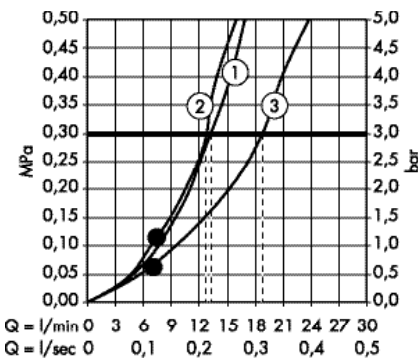
· Croma 100 Classic Ручной душ Multi # 28539000
