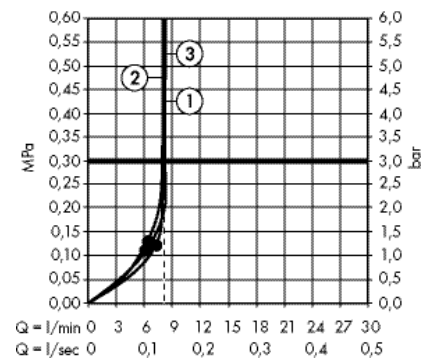
· Crometta 100 Ручной душ Multi EcoSmart 9 л / мин # 26826400
