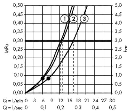
· Croma Select S Ручной душ Multi # 26800400
