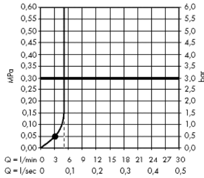
· Crometta Ручной душ 1jet Green 6 л / мин # 26334400
